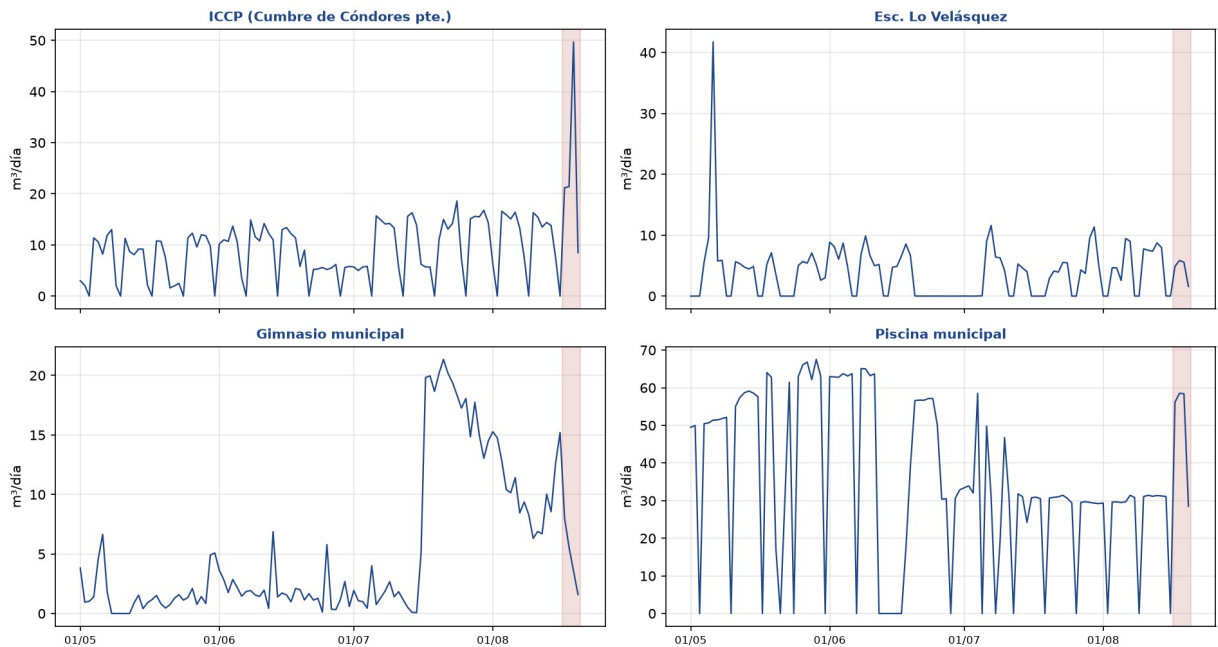
Consumo diario mayo-agosto 2026 (sombra = sin control WES)
